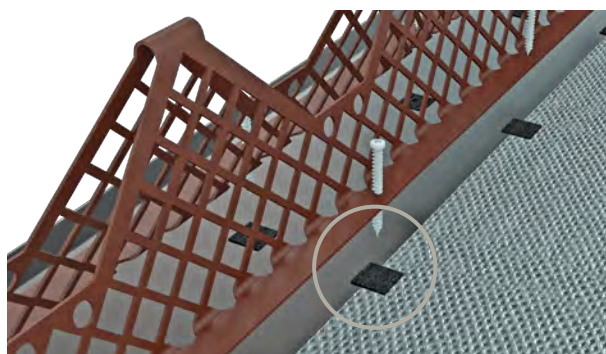
griglia di partenza parapasseri AC
