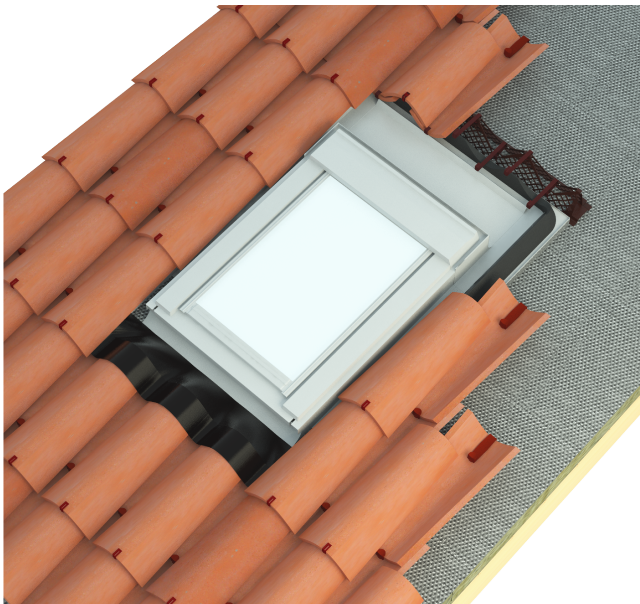
Vista del lucernario con il sistema AERcoppo®
