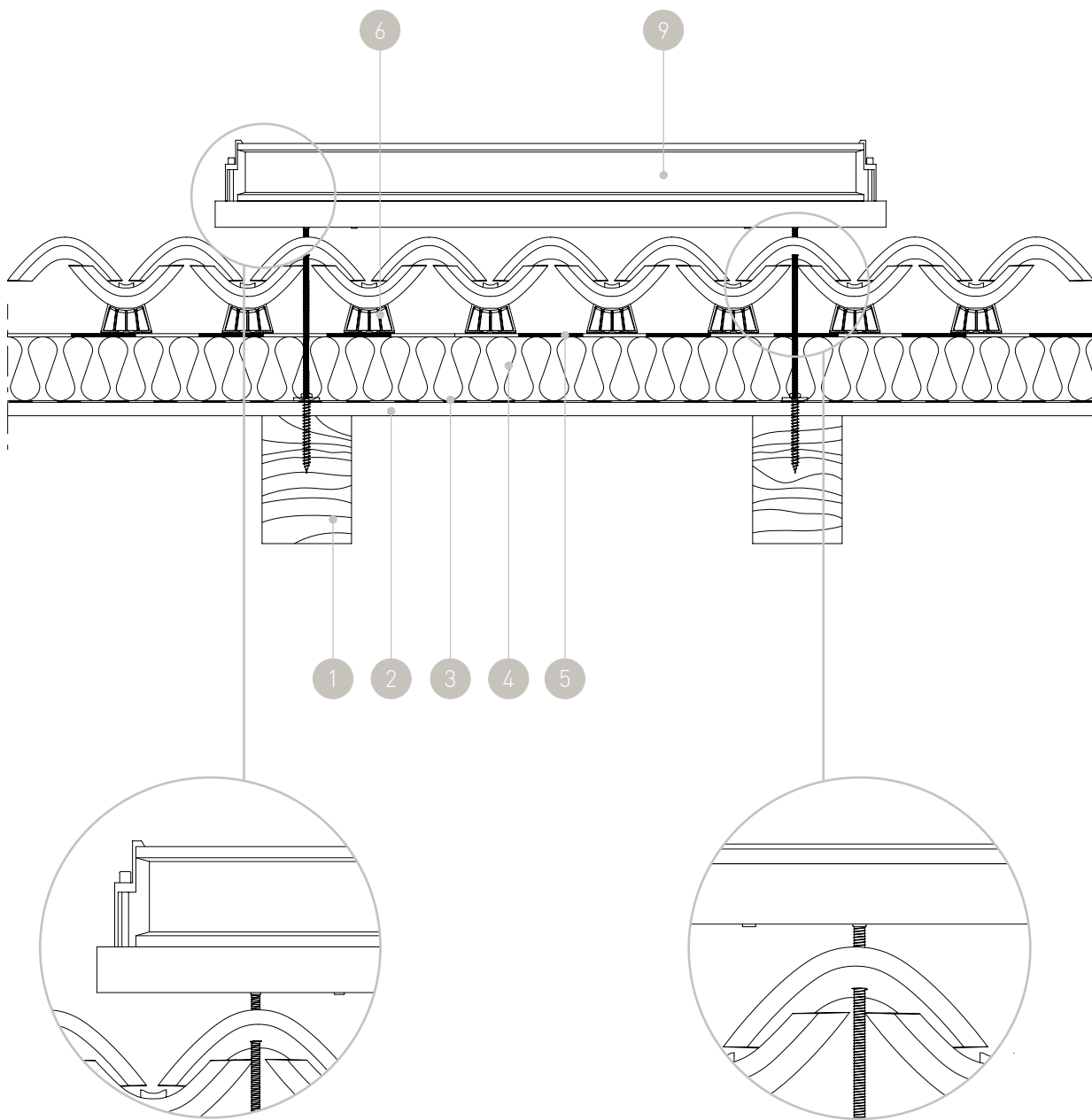
Installazione, con viti, della staffa di sostegno dei correntini metallici
