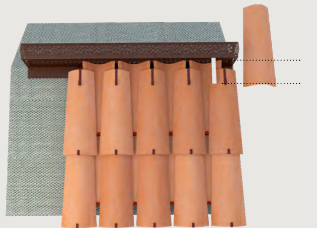
Taglio dell'ultima fila di coppi coperta
