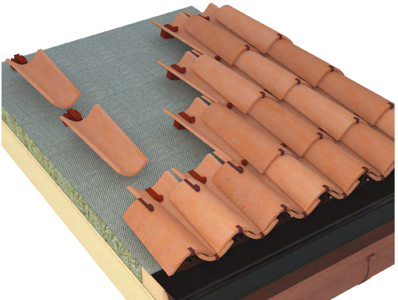
Vista dell'inserimento del Piedino AERcoppo® PC di rialzo ed ancoraggio dei coppi canale
