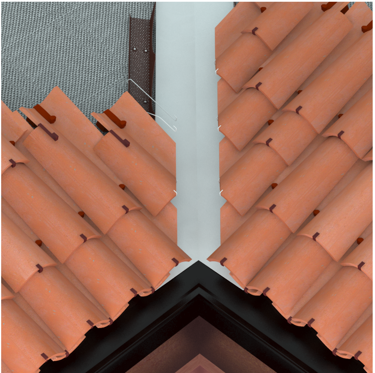
Particolare del compluvio in falda finito e griglie di compluvio CC
