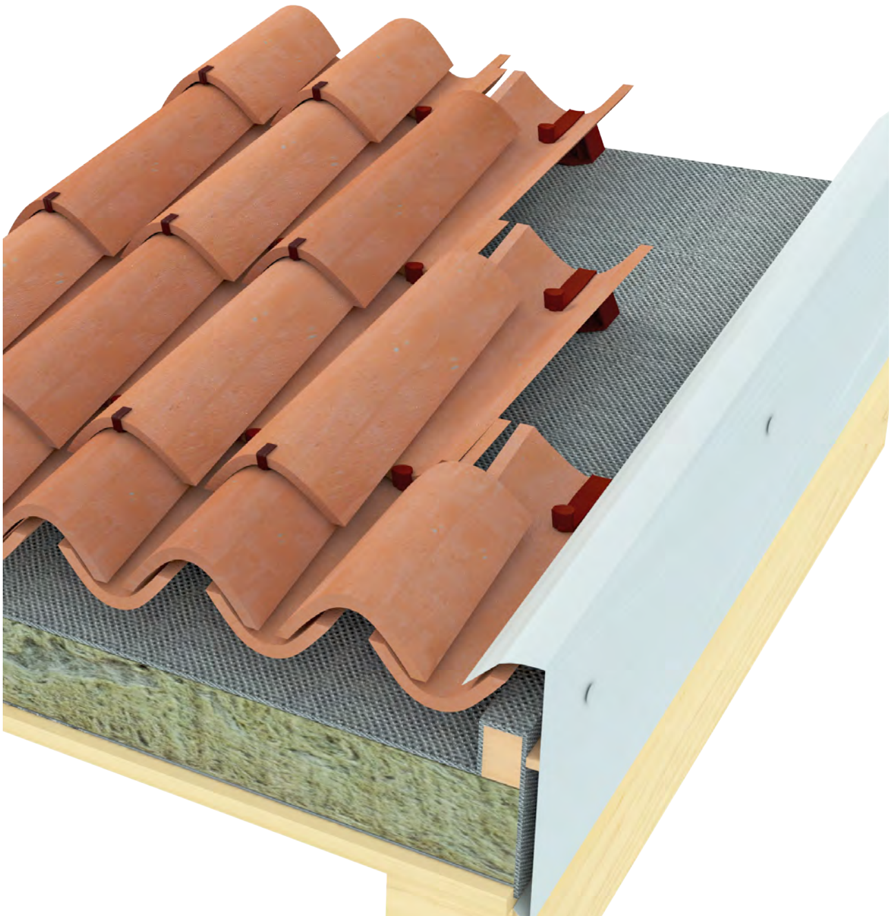
Vista della scossalina di chiusura laterale della falda
