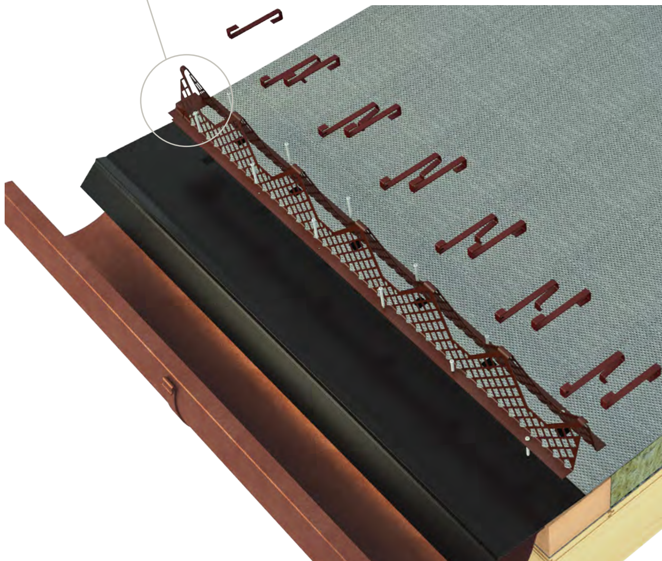
Vista dell'inserimento dei ganci G13 e G12 sulla griglia di partenza parapasseri AC
