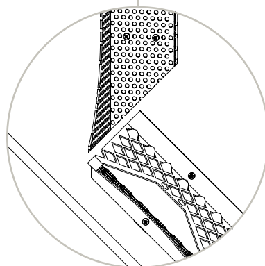
Particolare del raccordo tra la griglia di partenza parapasseri AC e la griglia di compluvio CC tagliata
