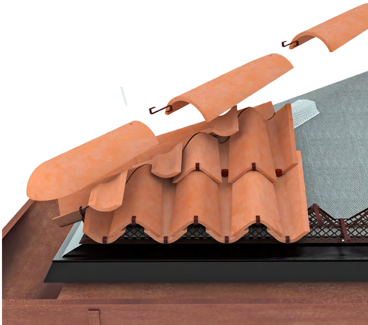
Particolare del displuvio in falda finito ed elemento di displuvio DCT
