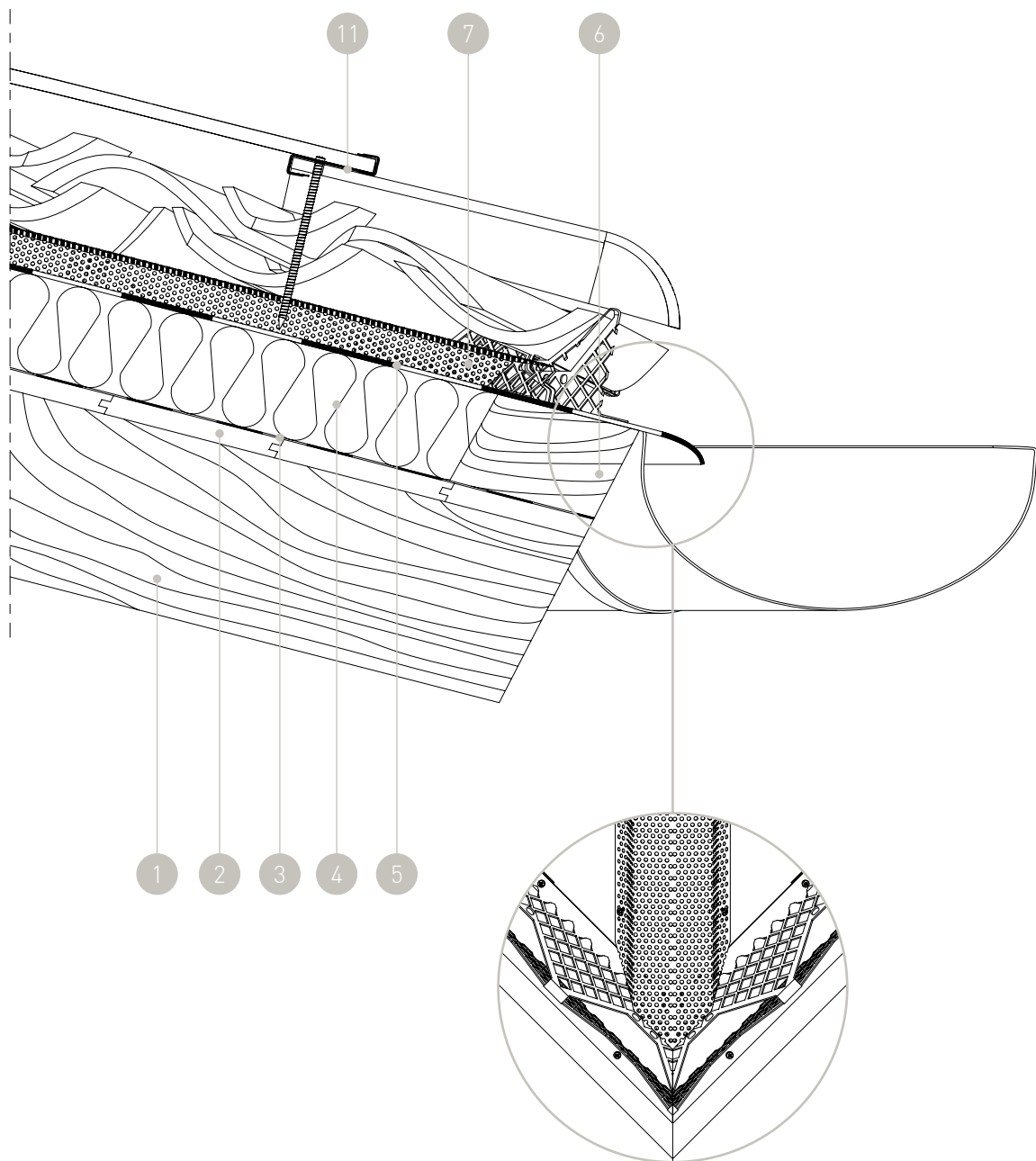
Particolare del raccordo tra la griglia di partenza parapasseri AC e l'elemento di displuvio DCT tagliato
